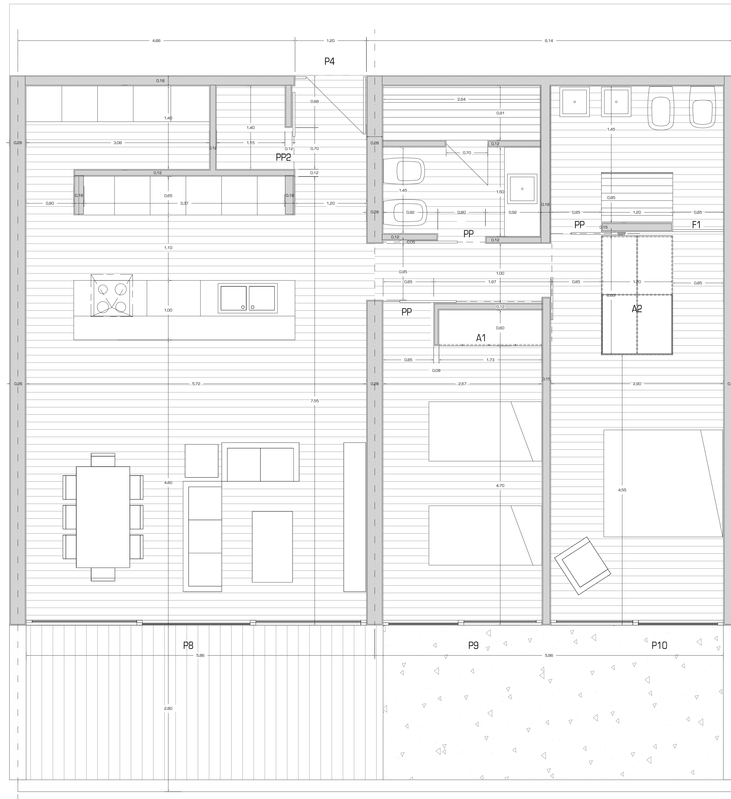
vivienda tipo 1
