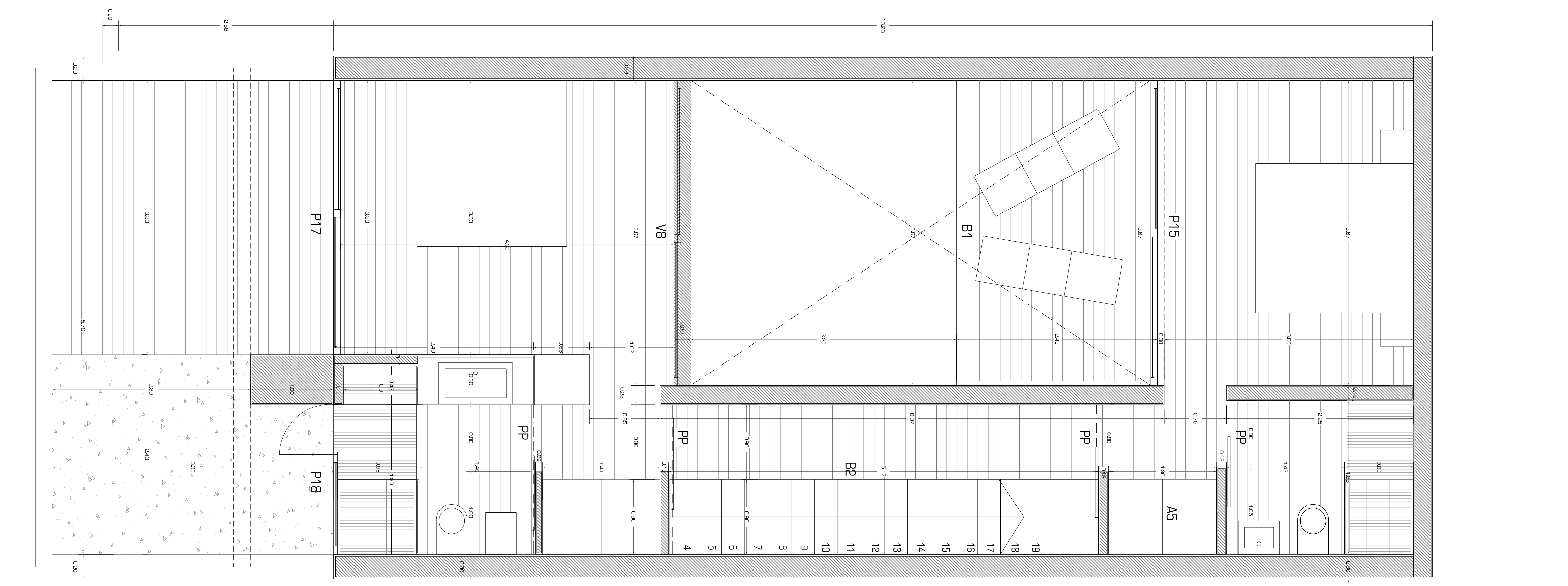
planta alta
